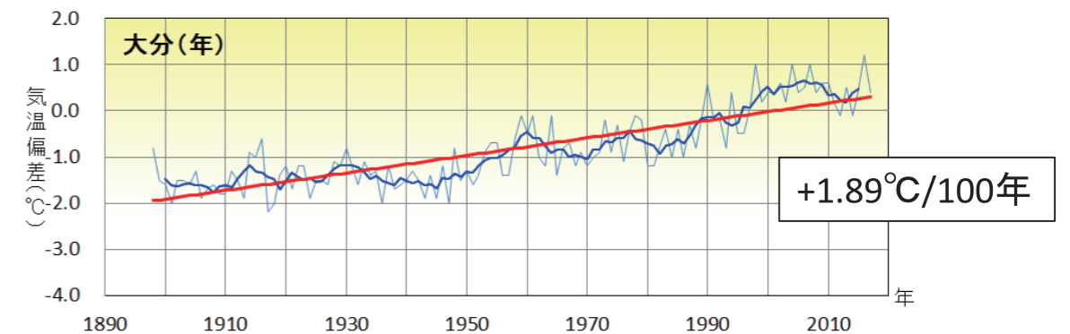
大分市の年平均気温の経年変化
