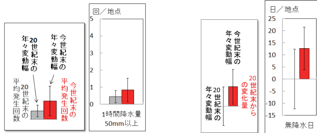
非常に激しい雨の年間発生回数の変化 (大分県)
