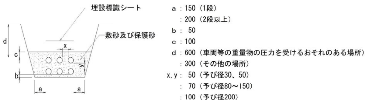
図－Ⅲ.11.1 管路式の地中埋設参考図
