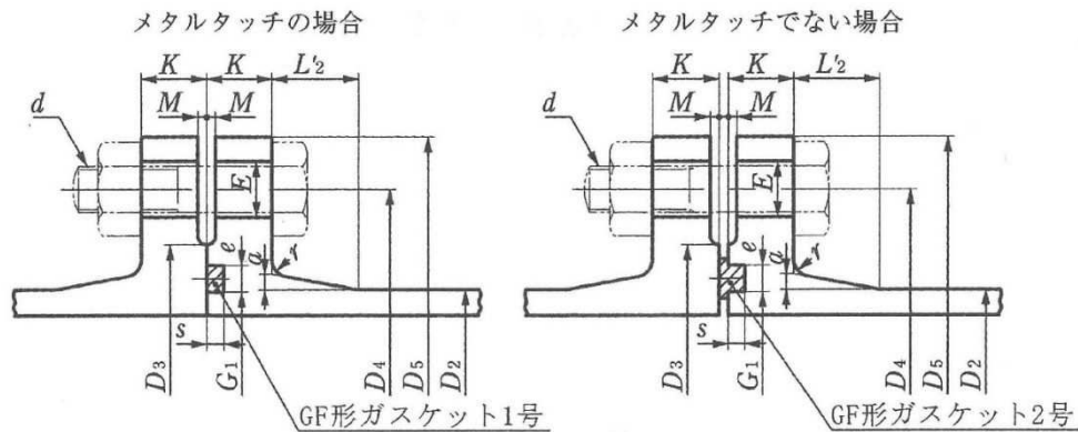
図ーⅡ.6.1 RF形（大型面座形）-GF形（溝形）フランジ
