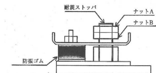
図－I. 3. 2 防振支持機器例
