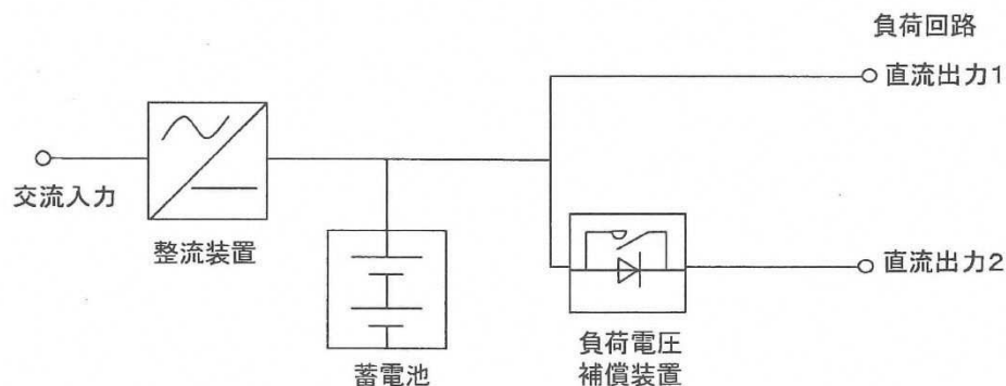
図一Ⅲ. 4. 1 直流電源設備システム構成の参考例
