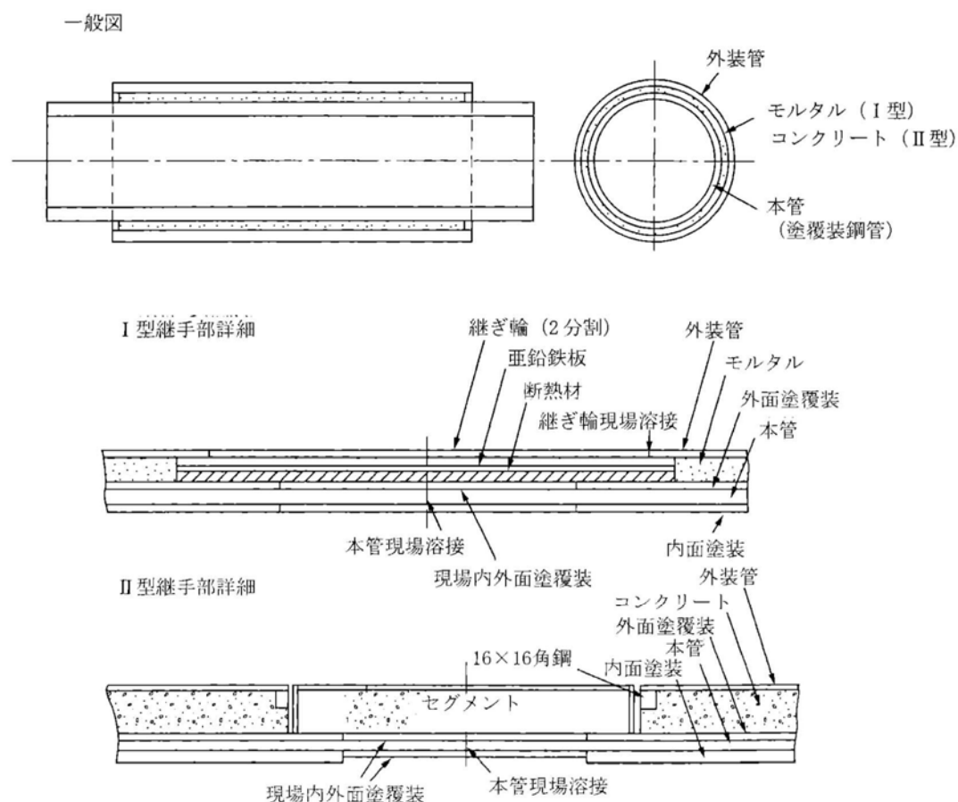
図－4.8.1 水道用推進鋼管
