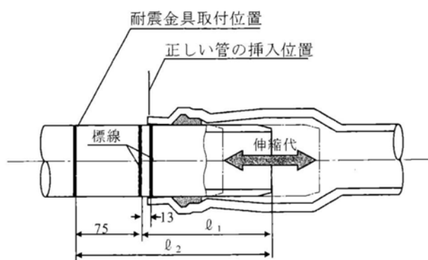
図-4.4.3 標線と管の挿入位置
