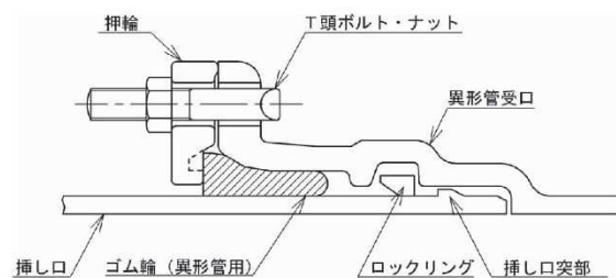
図－4.2.9 GX形異形管（呼び径75～450）
