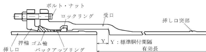
図-4.2.4 NS形直管（呼び径500～1000）
