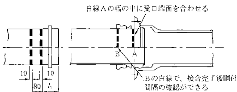
図-4.2.15 受口・挿し口の挿入完了（単位：mm）
