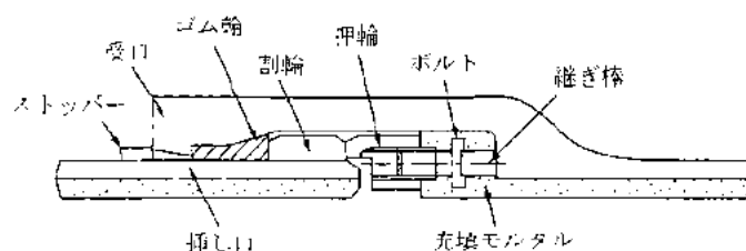
図-4.2.10 U形管の接合
