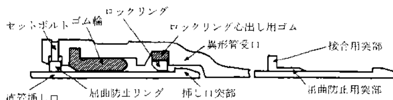
図-4.2.5 NS形異形管（呼び径75~250）
