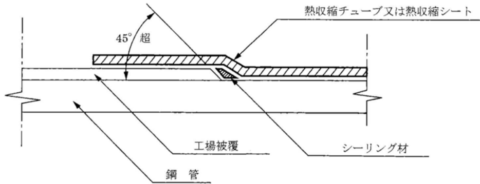
図-4.3.2 シーリング材の施工
