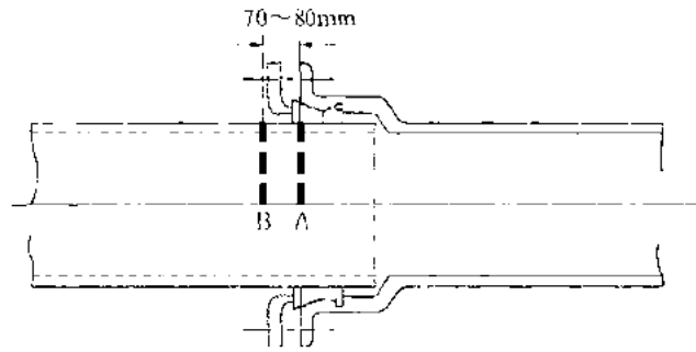
図-4.2.16 受口端面とB白線の端面側との間隔
