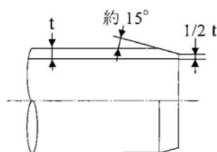
図-4.4.1 面取り
