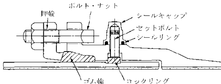
図-4.2.12 KF形管の接合
