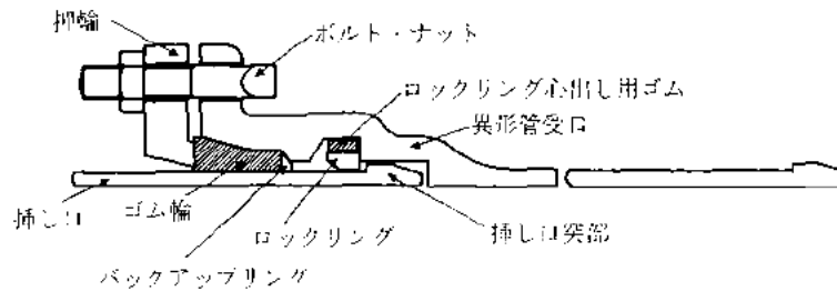
図-4.2.6 NS形異形管（呼び径300～450）
