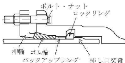
図-4.2.7 NS形異形管（呼び径500～1000）
