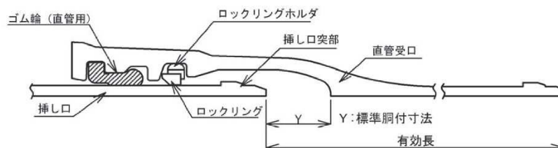
図-4.2.8 GX形直管（呼び径75～450）
