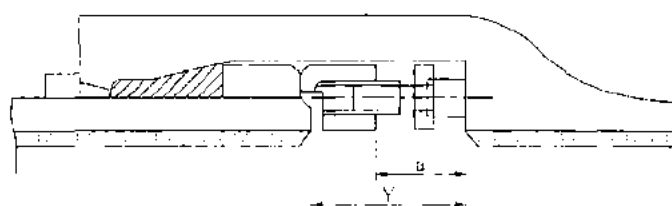
図-4.2.11 胴付間隔及び締付け完了時の押輪と受口底部の間隔
