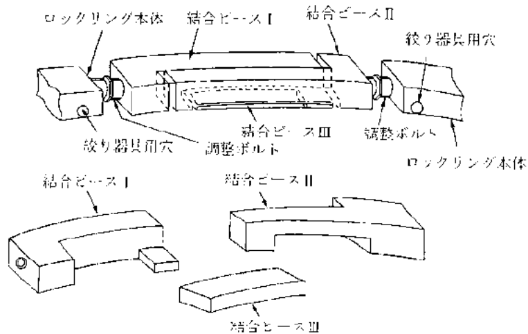
図-4.2.18 結合ピース・ロックリング接合部
