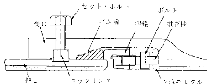
図-4.2.13 UF形管の接合
