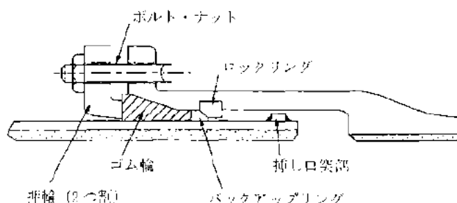
図-4.2.14 SⅡ形管の接合
