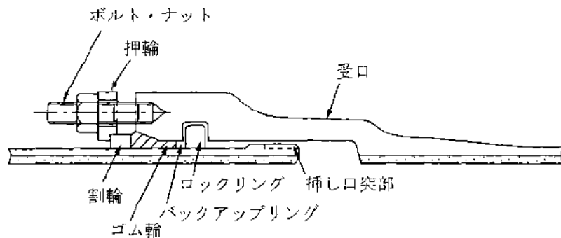
図-4.2.17 S形管の接合
