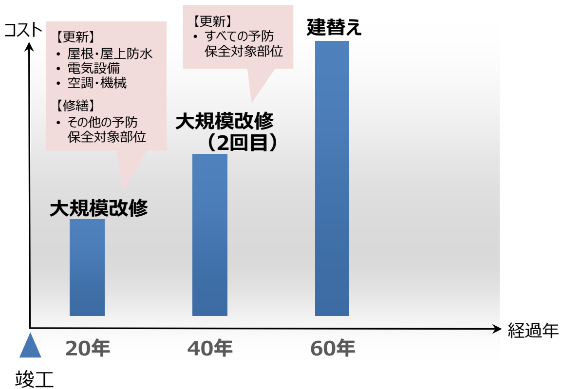
保全メニュー(鉄骨造)
