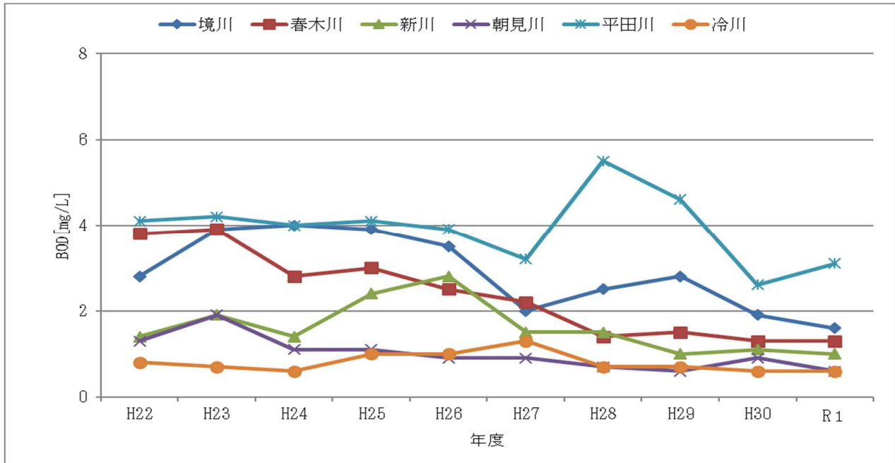
2.16 市内主要6河川のBOD濃度の各年度の経年変化
