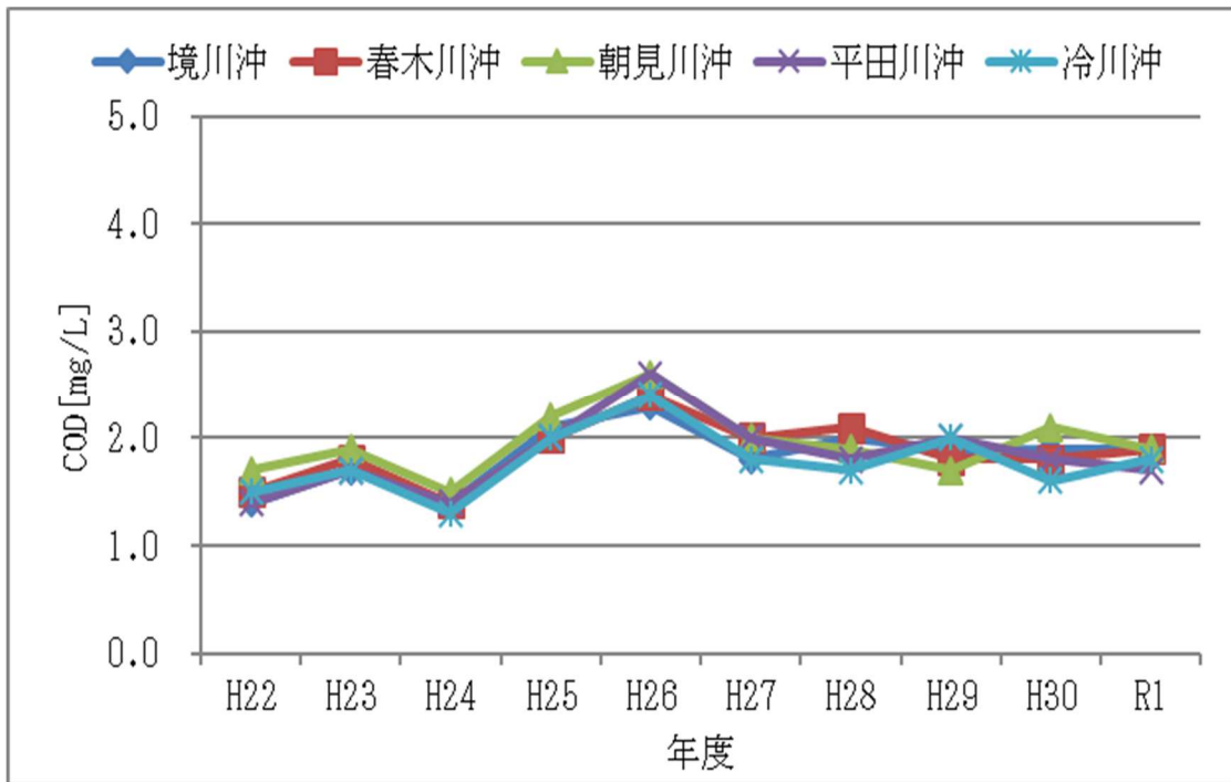
図表 2.17 別府湾地先海域 5 定点の COD 濃度の各年度の経年変化
