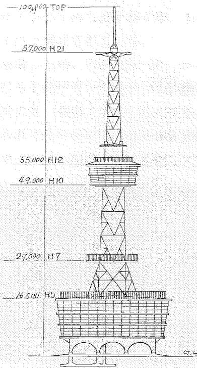
正面略図
