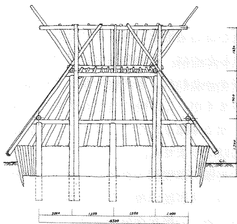
竪穴式住居断面図
