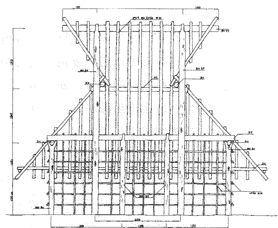
平地式住居断面図
