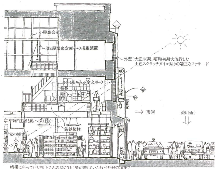
吹抜け廻り断面図
