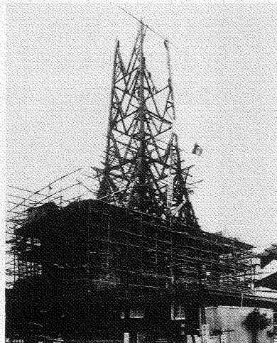
タワー鉄骨組上げ
