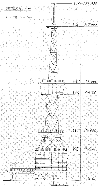
側面略図
