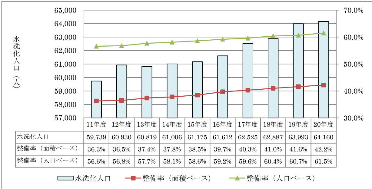
図表 3.11 下水道整備率の年次推移（各年度末現在）
