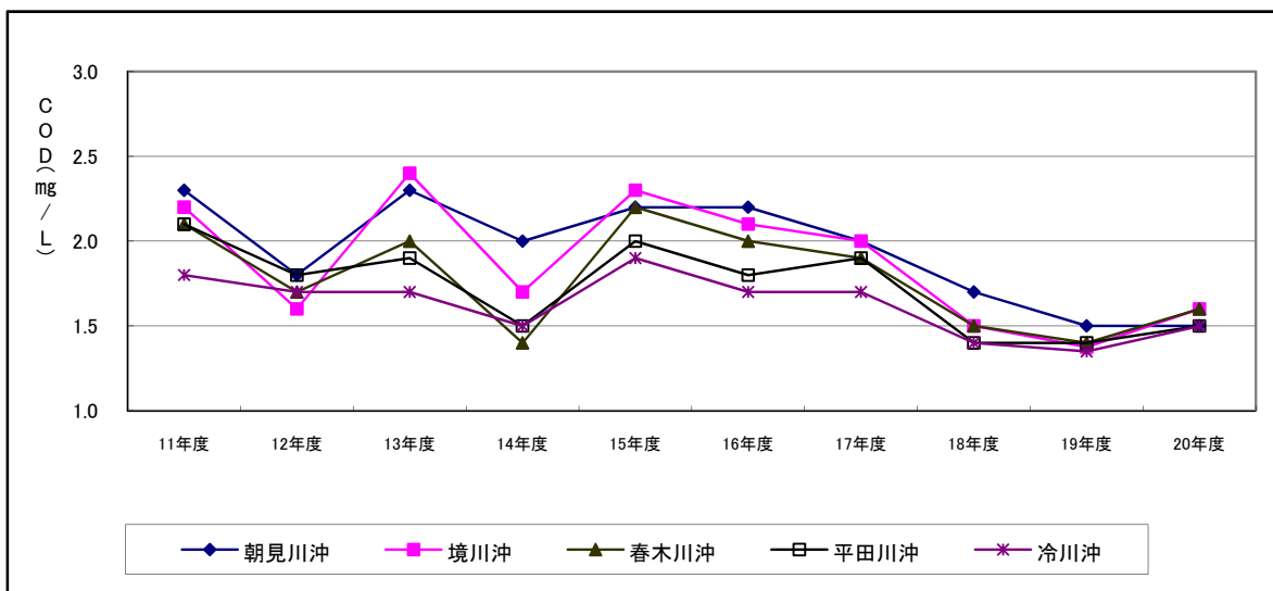
図表 3.14 別府湾地先海域5定点のCOD濃度の各年度の経年変化
