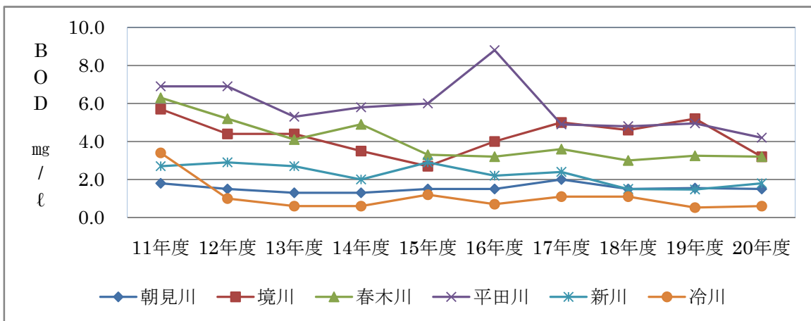
図表 3.13 市内主要6河川のBOD濃度の各年度の経年変化
