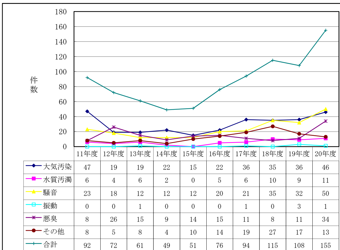
図表 3.8 過去10年間の公害苦情件数の推移（平成18年度の「その他」に土壌汚染1件を含む）
